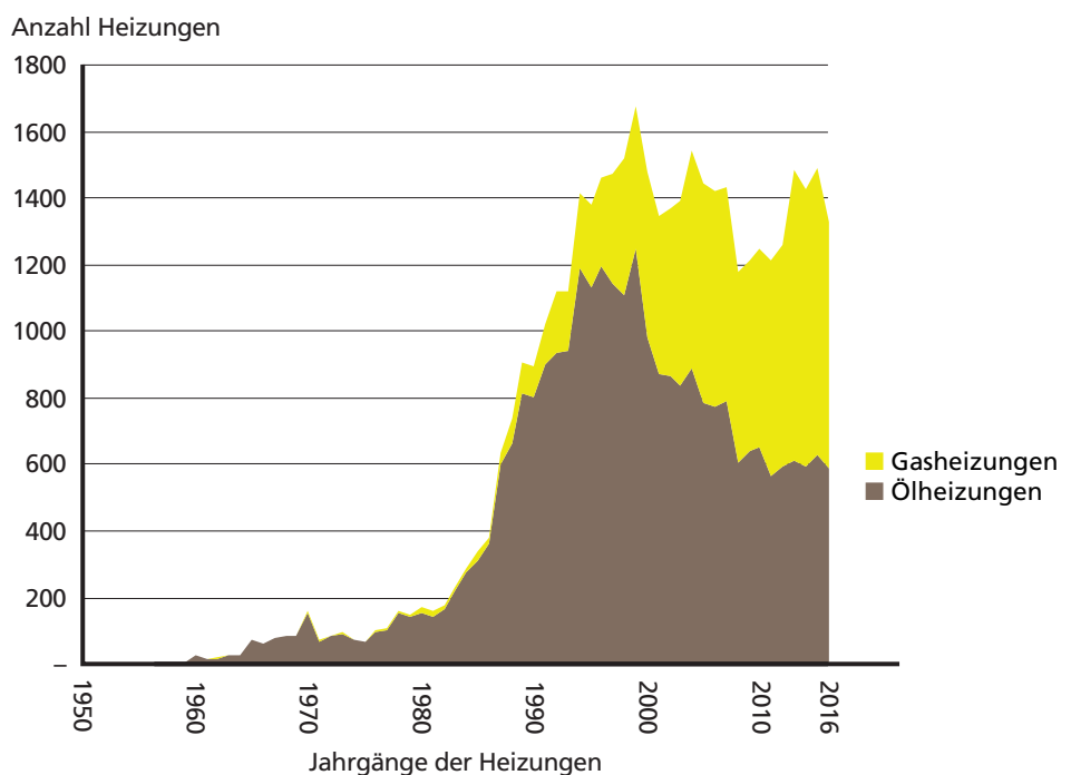
Abbildung 7 Altersstruktur Öl- und Gasheizungen im Kanton Solothurn
