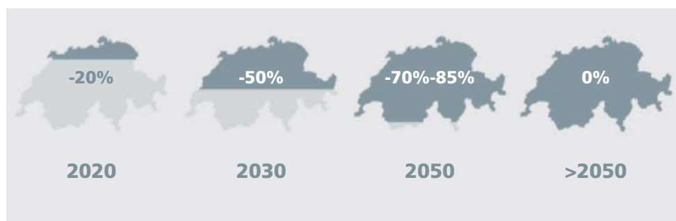
Abbildung 1 Nationale Emissionsreduktionsziele in der Schweiz (im Vergleich zu 1990)
