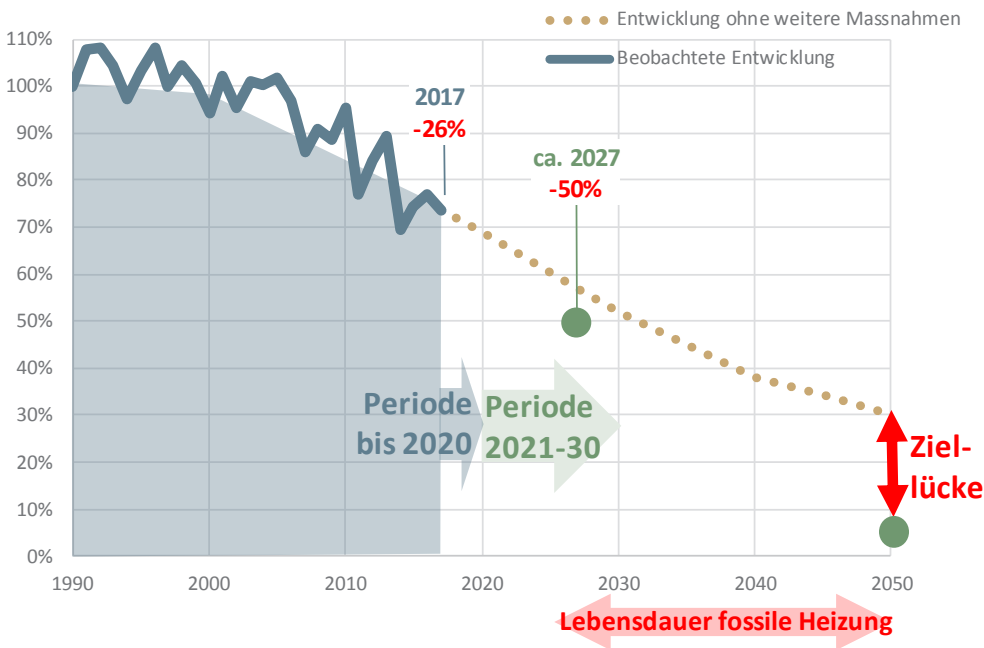
Abbildung 8 CO 2 -Zielerreichung: Je nach langfristiger Zielsetzung ergibt sich eine deutliche Ziellücke
